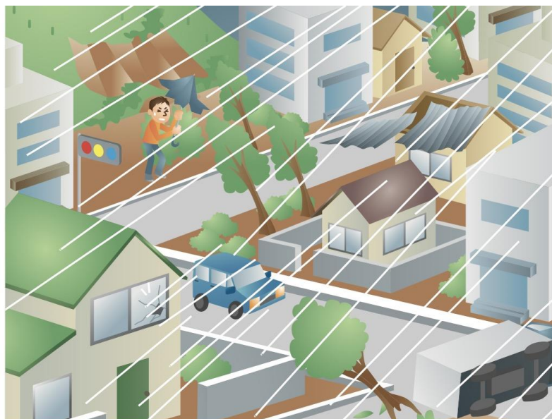
图 4 台风或飓风
