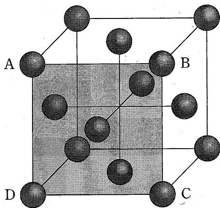
図2 アルミニウムの単位格子
