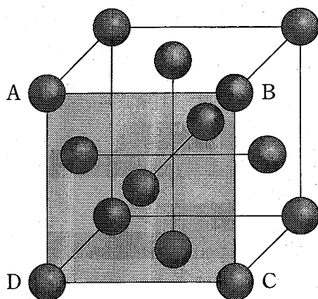
図2 アルミニウムの単位格子
