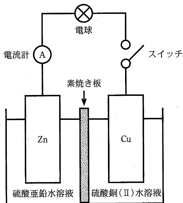
図1. 電池の概略図
